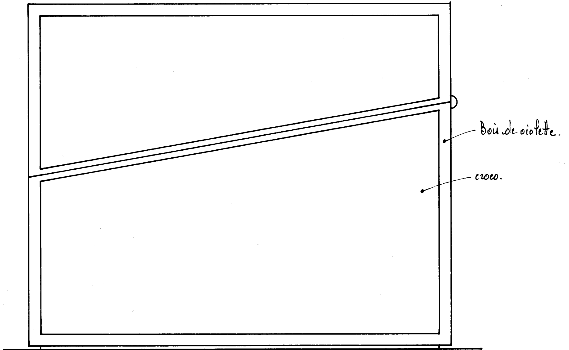
.. ÉCRIN m BACCARAT. 210 x 183 x 148 MM. VUE DE COTÉ. ATELIER SANSON. 03. 2018.
